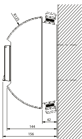
BOČNÍ POHLED
